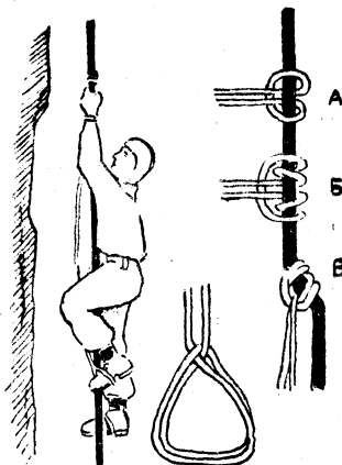
«Петли Пруссика» 71
